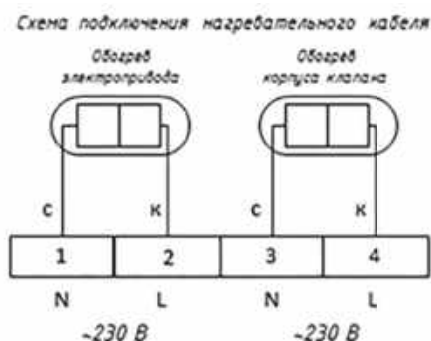
Клапан противопожарный обратный КПВ.01(02;03)...-ОМС прямоугольного сечения
